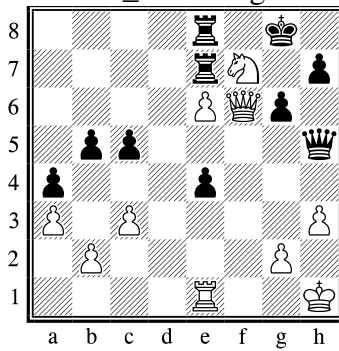
mat1_15: Qf6-h8
