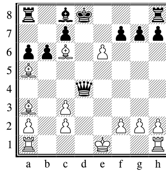
mat1_16: e6-e7
